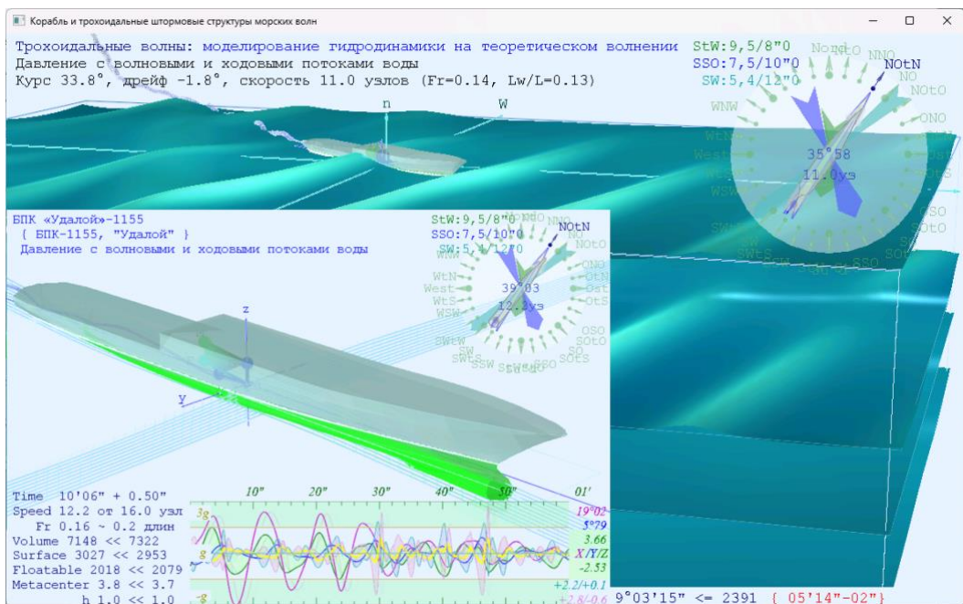
Рис. 10. Изображение всех волновых полей, корабля и маршрута его движения для наглядного представления хода вычислительного эксперимента. В верхних строках записываются действующие режимы моделирования морского волнения и гидромеханики корабля. В нижней строке текущее компьютерное время и количество выполненных циклов. Красные отсчеты минут означают нехватку вычислительных ресурсов, и отставание вычислительного эксперимента от требуемого реального времени.
