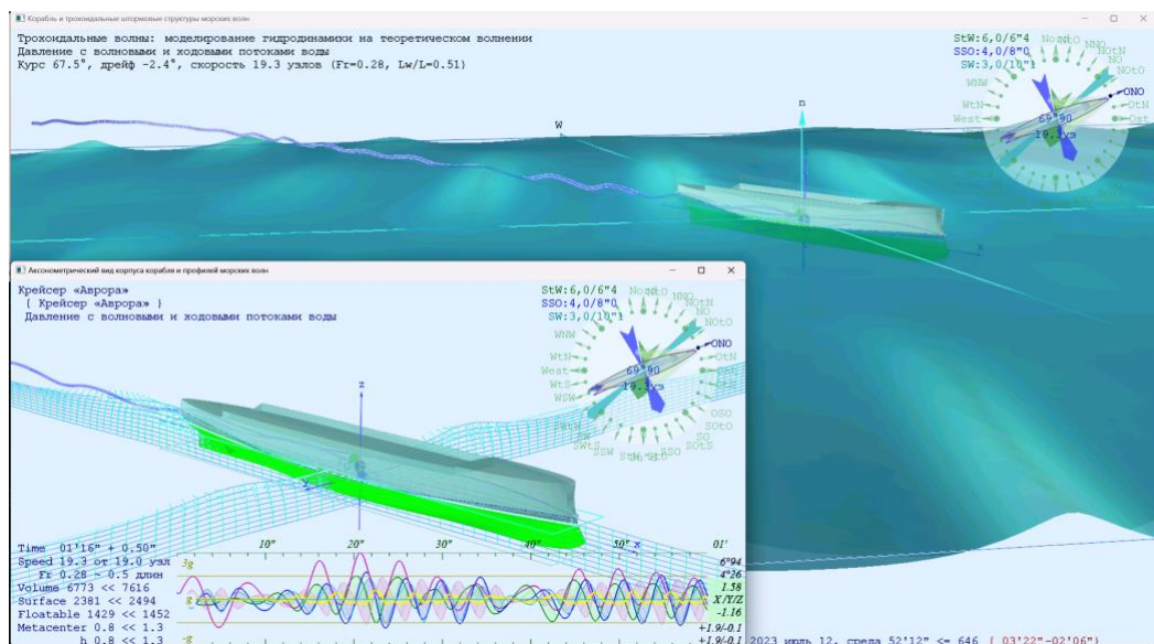
Рис. 9. Прорисовки динамического состояния корпуса корабля. Справа сверху картушка с действующим и заданным курсом корабля. Стрелками показаны длина, крутизна и направления движения групповых структур волн. В нижней части экрана графики бортовой, килевой и вертикальной качки, с вертикальными ускорениями в средней части корпуса и в оконечностях.
