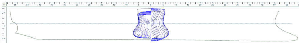
Рис. 11. Вариант экспорта модели корабля для работы в DesignCAD-express (*.dc2) в традиционном «бумажном» представлении теоретических чертежей. Здесь разметка аппликат приводится к основной линии.
