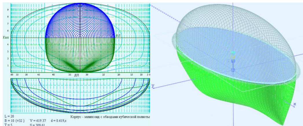
Рис. 4. Выбор варианта простейшего «Корпуса» с однократным улучшением скуловых обводов по алгоритму: « обводы скуловых волн ».
