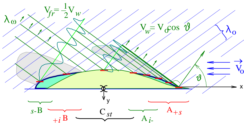
Рис. 7. Волнообразование, как процесс отражения волн от поверхности корпуса корабля. В зонах A_{+s} и s-B происходит рост гребня трохoidalной волны, неспособной оторваться от корпуса судна.
