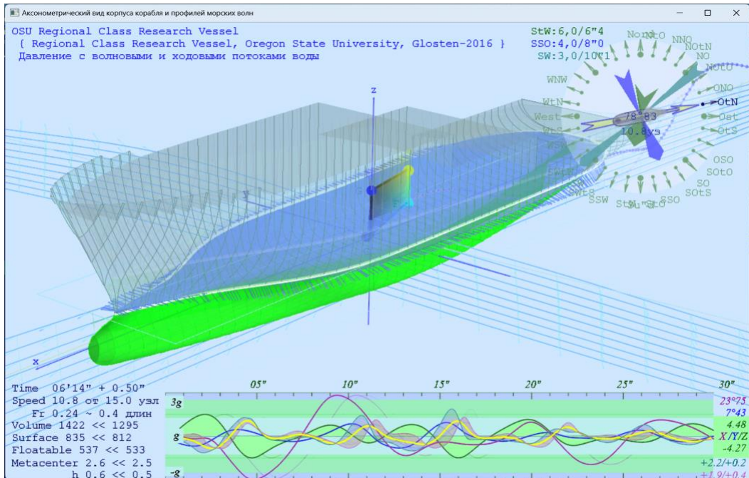
Рис. 13. Ход вычислительного эксперимента в окне для представления гидромеханики корабля. По траектории движения центра корабельного базиса видна вертикальная качка и сильный дрейф в моменты экстремальной бортовой качки. Внизу графики бортовой X , килевой Y и вертикальной Z качки с масштабной шкалой справа. На левой шкале масштаб для кривых вертикальных ускорений.
