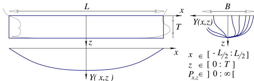
Рис. 5. Размещения аналитической модели формы корпуса корабля
