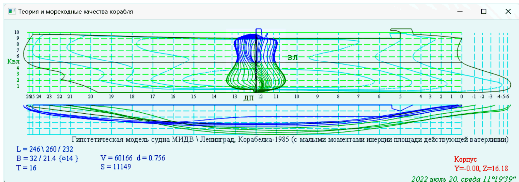
Рис. 3. Образцовая экспериментальная модель корпуса гипотетического корабля с уменьшенными моментами инерции площади действующей ватерлинии (МИДВ), и со смещенным в нос центром величины подводного объема. В 1985 г. модель участвовала в мореходных испытаниях [1] в опытовом бассейне кафедры теории корабля Ленинградского кораблестроительного института под руководством профессора Александра Николаевича Холодилина
