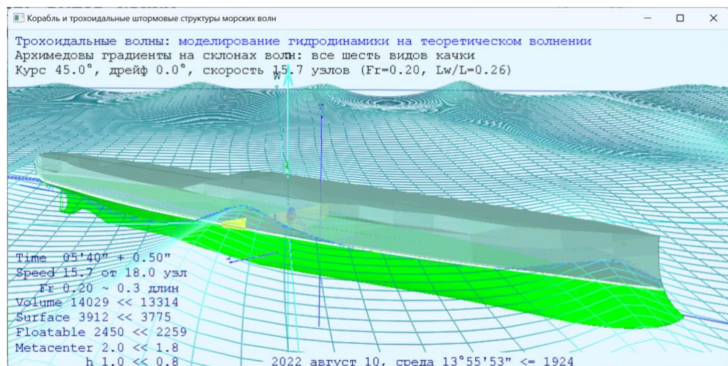
Рис. 14. «Корабль и трогоидальные штормовые структуры морских волн» – воспроизведение морского волнения в опытовых изысканиях мореходности корабля в условиях штормового плавания. Контурные прорисовки профилей трогоидальных волн большой крутизны выполняются на фоне соизмеримой по высоте длиннопериодной зыби.
